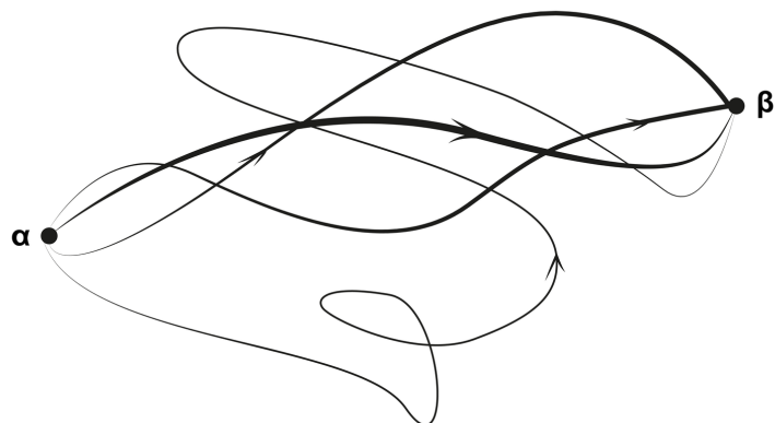
Obr. 1: Na těchto čtyřech grafech označuje \alpha zdroj částic nebo počáteční bod, \beta je bod na obrazovce označující místo, kam částice dorazí. První graf
